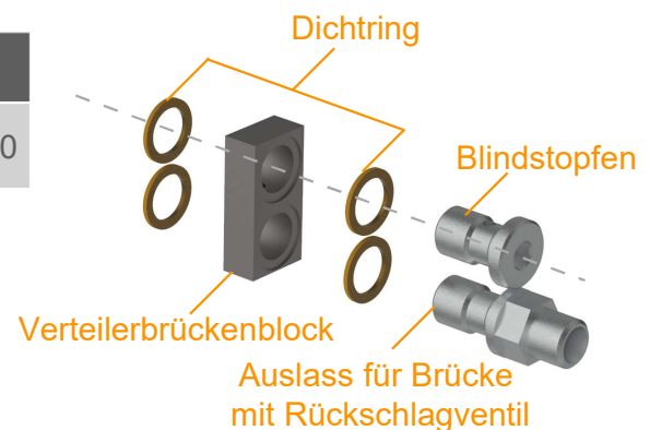
Abb. 18.2 Verteilerbrücke mit Auslass und Rückschlagventil
