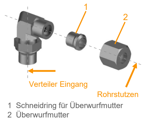
Abb. 12.2 Winkel-Einschraubverschraubung
