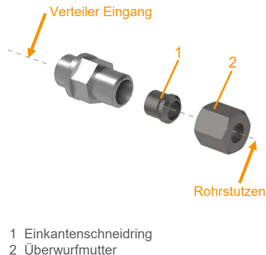
Abb. 12.1 Gerade Einschraubverschraubung
