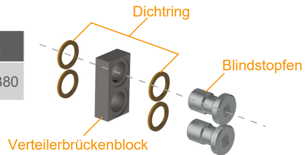
Abb. 18.1 Kit-Verteilerbrücke ohne Auslass
