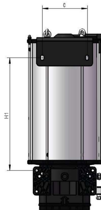
Abb. 19.3 Anschlussmaße (Oben) für ALPB HSC-AC Pumpe (Rührflügel) für 15L und 20L Pumpe
