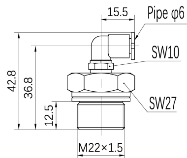
Abb. 18.1 Anschlussverschraubung bei einem Bypass
