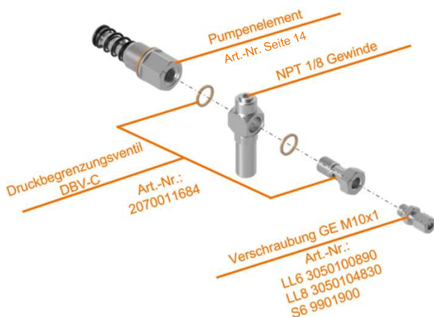
Abb. 16.2 Explosionszeichnung PE mit gerader Verschraubung
