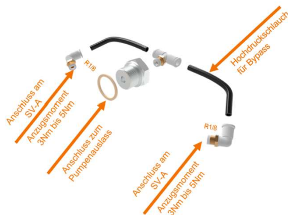
Abb. 18.6 Zweiseitiger Bypass Kit
