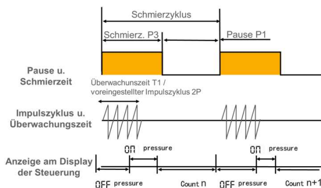
Abb. 25.3 T1 < 3P
