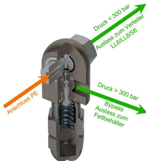
Abb. 17.1 DBV-A Funktionsprinzip
