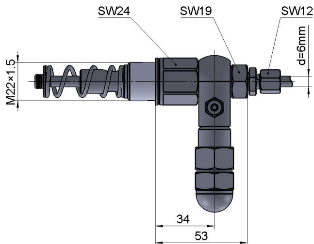
Abb. 17.3 Abmessungen DBV-A mit montiertem Pumpenelement PE
