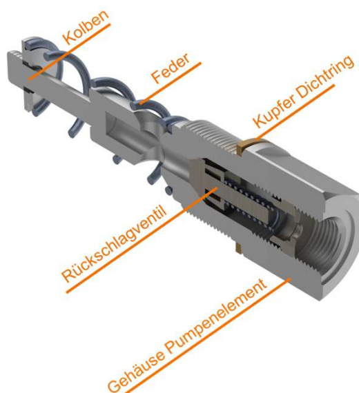
Abb. 14.2 Pumpenelement Aufbau
