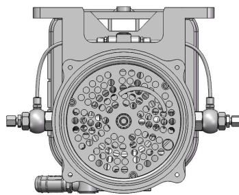
Abb. 18.3 Pumpe mit zwei Bypässen u. zwei DBV-A
