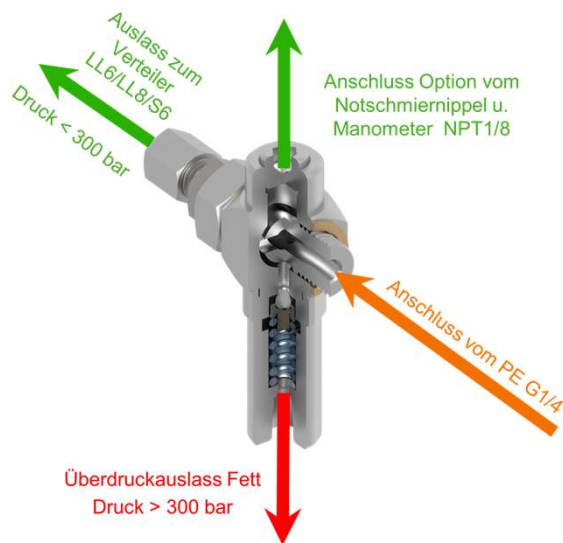
Abb. 16.1 DBV-C Funktionsprinzip
