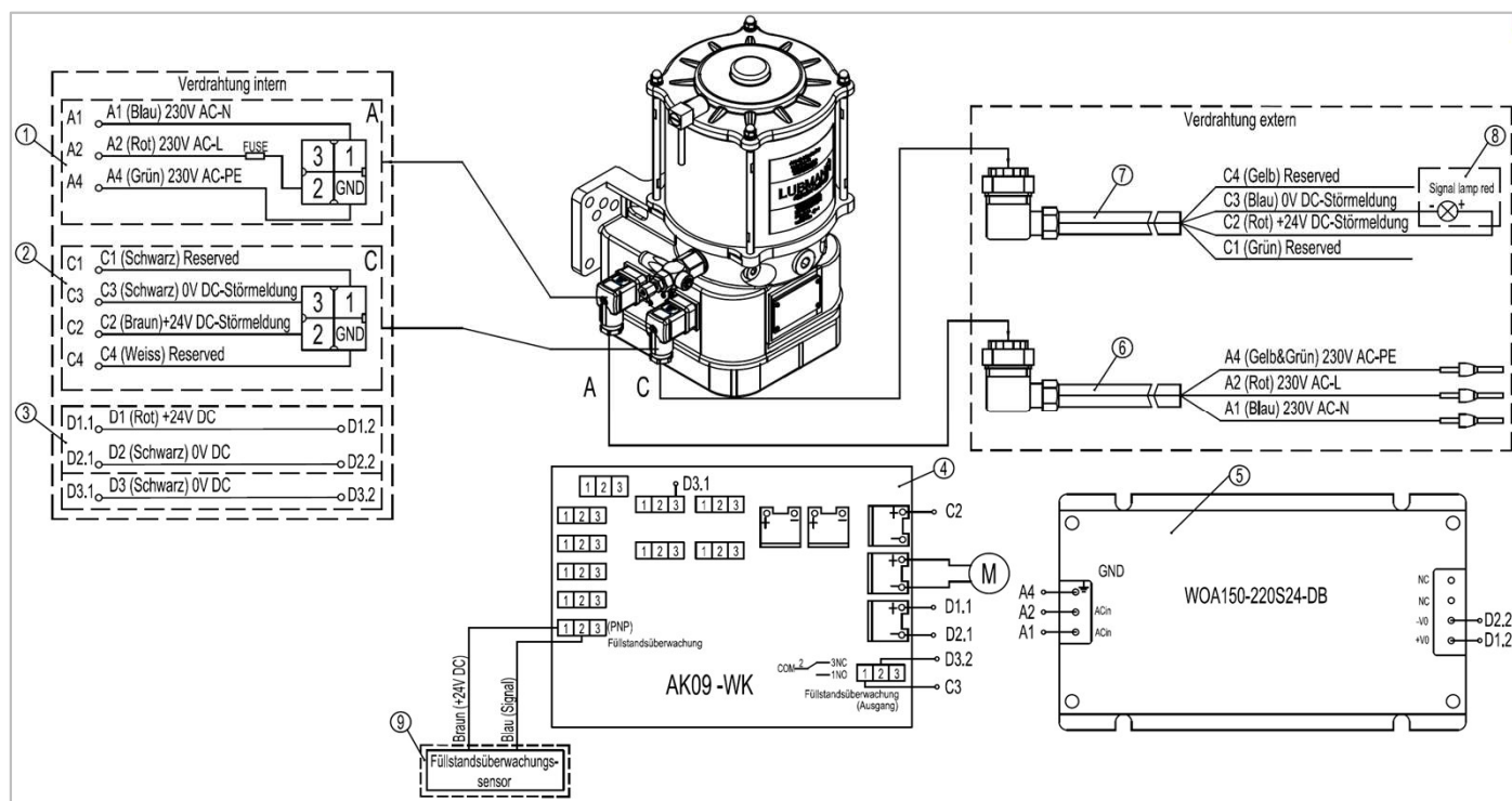
Abb. 27.1 Steckerbelegung für ALPB-HSC-AC ohne Steuergerät
