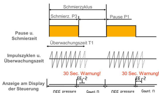
Abb. 25.4 T1 > 3P
